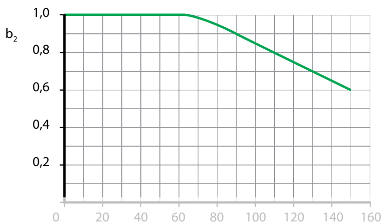
Fattore temperatura b_2 per superfici di strisciamento acciaio/tessuto PTFE Temperature factor b_2 for steel/PTFE fabric sliding contact surface combination
